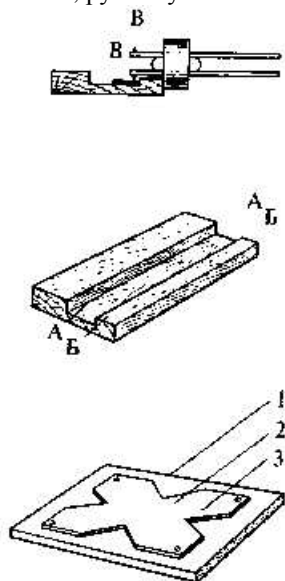
59. Резка штапиков и треугольных фигур
