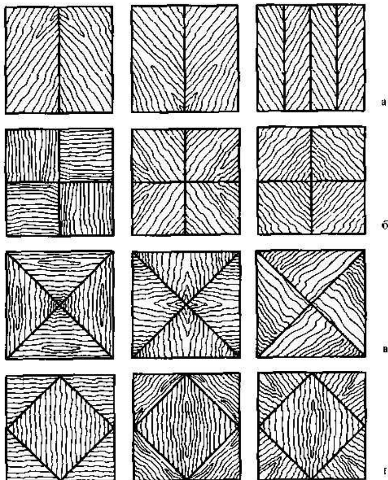
60. Виды декоративного фанерования:
