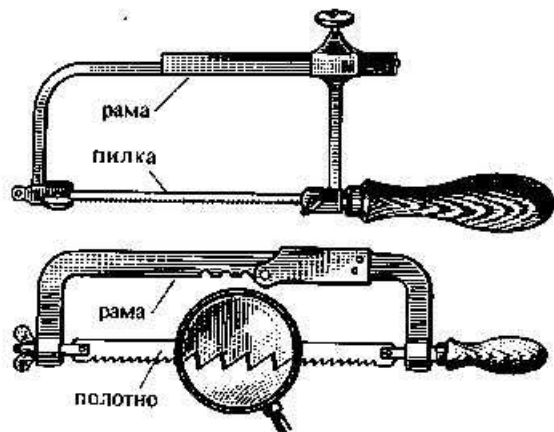
55. Слесарный лобзик Слесарная ножовка
